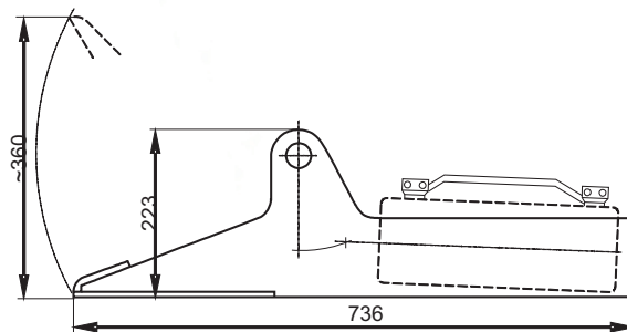
DźWIGNIK RAMIENIOWY
