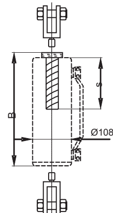
DźWIGNIK DWUSTRONNEGO DZIAŁANIA
