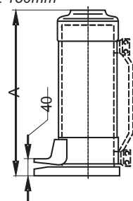
DźWIGNIK BOCZNIE PODNOŚĄCY
